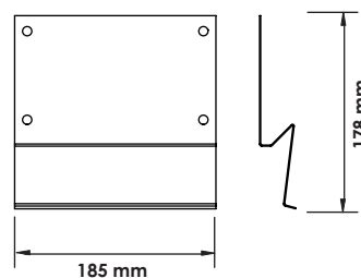
08-003-03 BRACKET F. 4 WAY WIELAND
